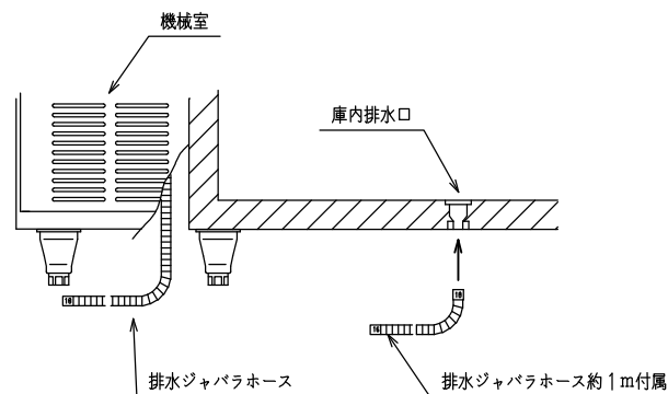
排水部詳細
