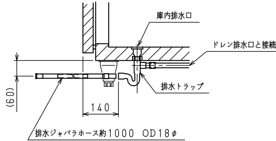
排水部詳細
